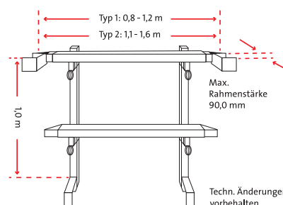
Skizze FENSTER-ABSTURZSICHERUNG
